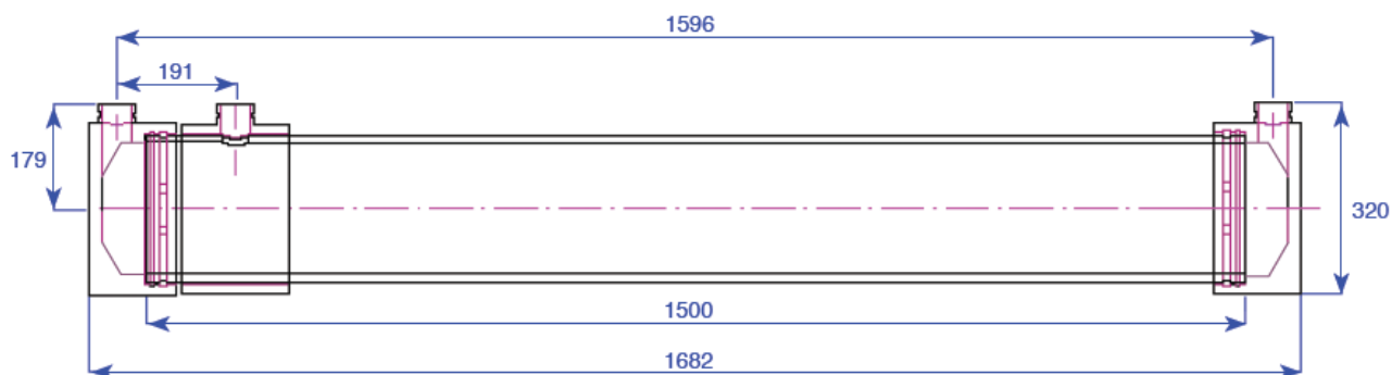
Рис. 2: Габаритные размеры ZW700B-10060 с торцевыми крышками (мм)
