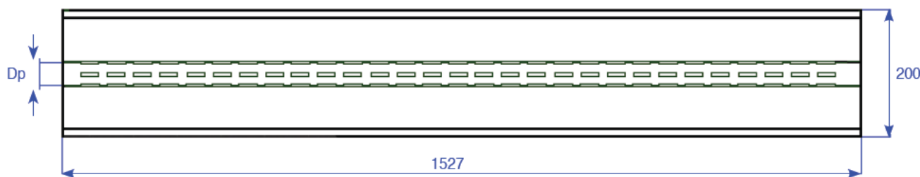
Рисунок 2: Габаритные размеры ZW700B-8060X (мм)
