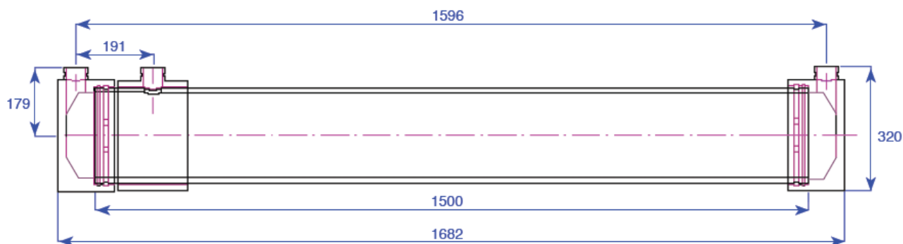
Рисунок 2: Габаритные размеры ZW700B-10060 с торцевыми крышками (мм)
