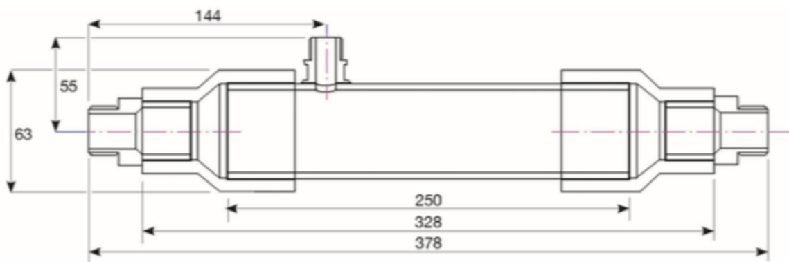
Рисунок 2: Габаритные размеры ZW700B-225
