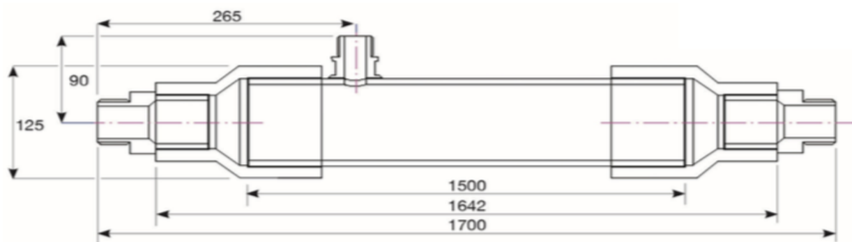
Рисунок 2: Габаритные размеры ZW700B-4150
