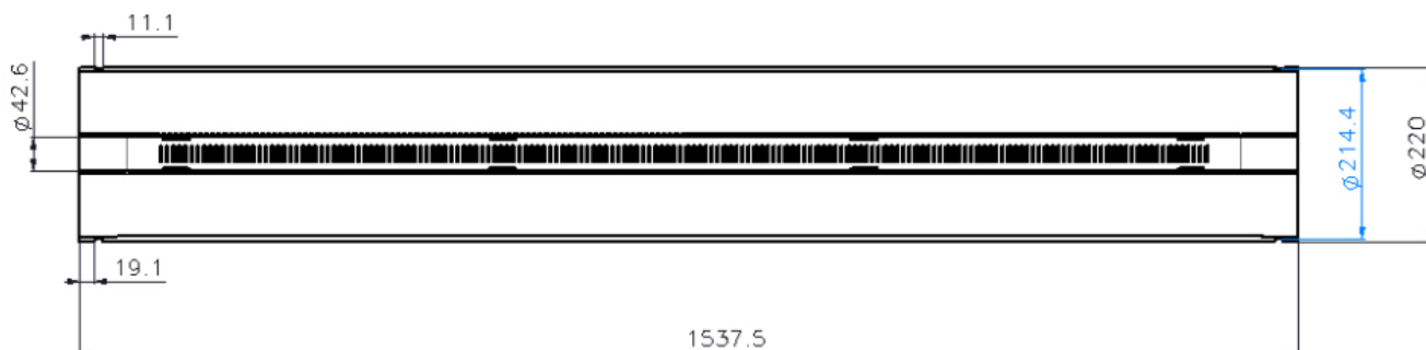
Рисунок 2: Габаритные размеры ZW700B-9060 (мм)
